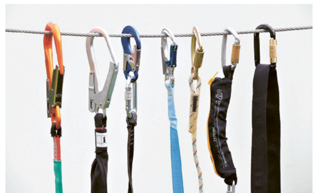
12 Sicherheitskarabinerhaken verschiedener Art.
