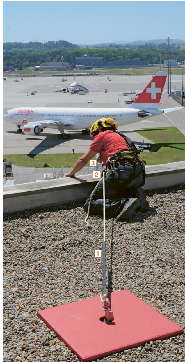
13 Auf einem Dach arbeitende Personen, die durch Auffanggurten an einem Sicherungsseil gesichert sind. Die Länge des Sicherungsseiles lässt sich mit einem festklemmenden Seilkürzer einstellen. Er ist so eingestellt, dass die gesicherte Person den Dachrand gerade noch erreichen kann.
