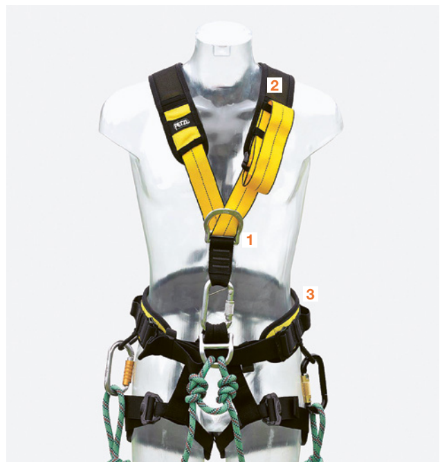
4 Komplettgurt (EN 361 und EN 358).
